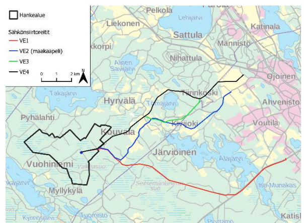
Niinimäen tuulivoimahankkeen alue ja eri suunniteluvaihtoehdot sähkönsiirtoreiteille. Kuva: Myrsky Energia Oy
